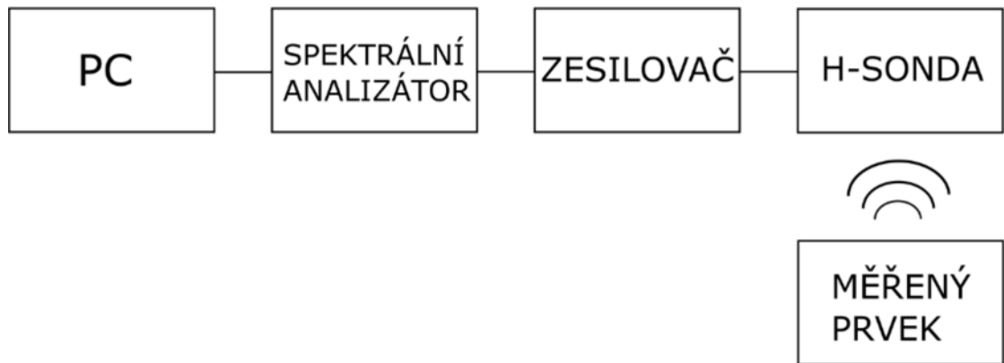
obr. 21: Blokové schéma měřicí sestavy
