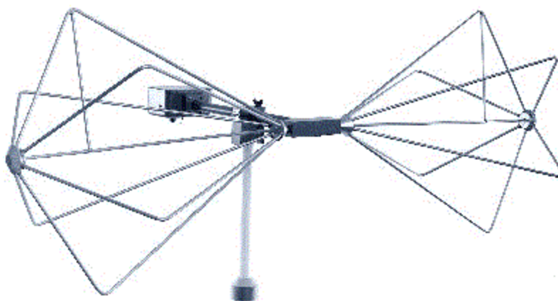
obr. 5: Bikónická anténa [2]
