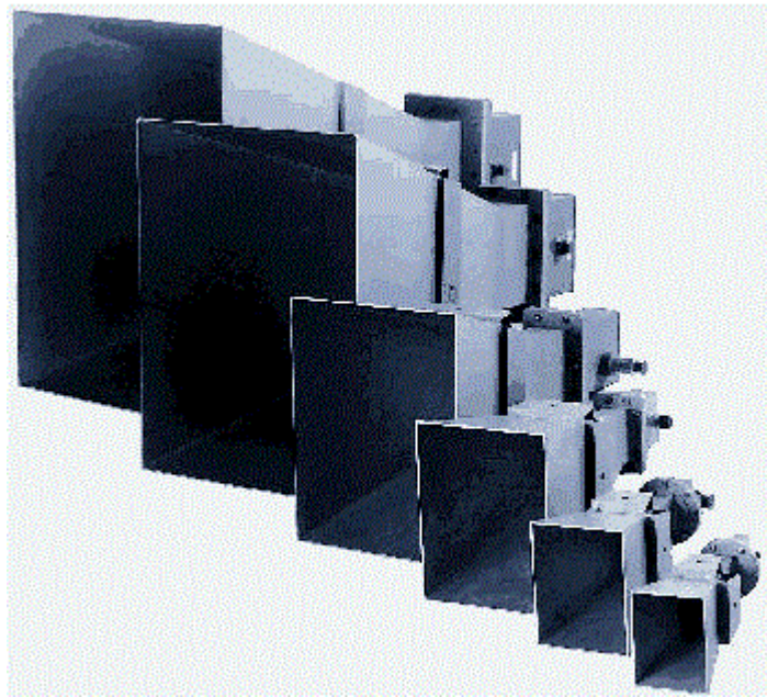
obr. 8: Trychtýřová anténa [2]
